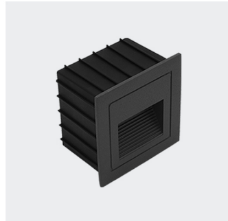
GQ1571 Lamp:LED 1×3W Size:90×90×55
